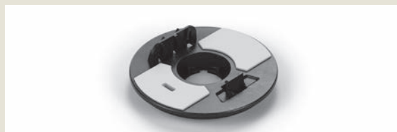
Tête UNIVERSALE autonivelante ø 110 mm pour lambour- des en aluminium et en bois Selbstnivellierender UNIVERSAL-Kopf ø 110 mm für Alu- Holz-UK
